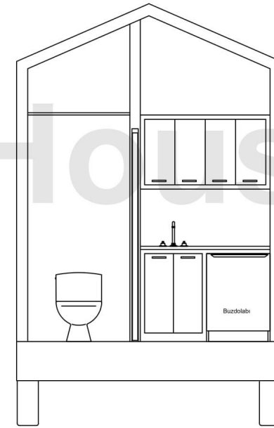
Mutfak ve Banyo Enkesiti
