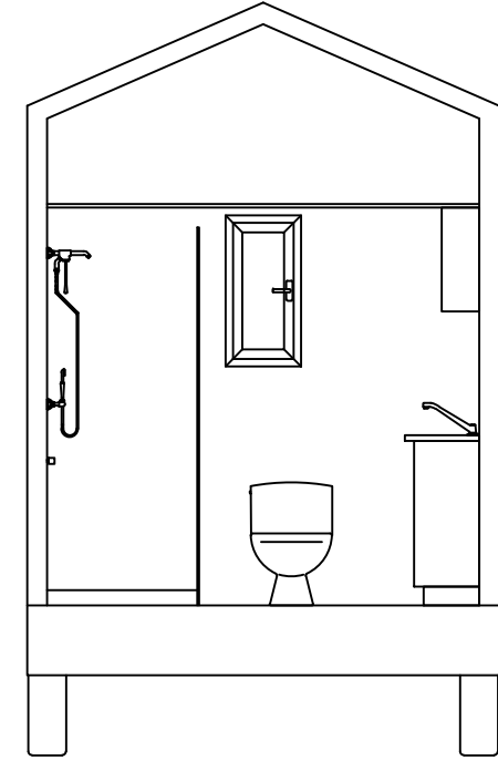
Banyo Enkesiti
